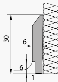
OP30RB CLEAN ROOM MET UITSPARING
