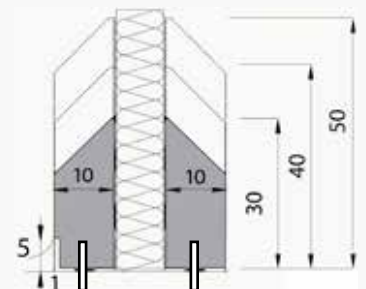
IP 30-40-50RB MET UITSPARING OF R RECHT
