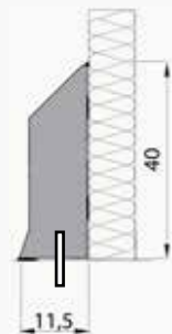
IP 30-40-50RB MET UITSPARING OF R RECHT
