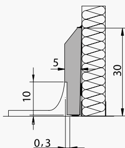
OP30RB CLEAN ROOM MET UITSPARING
