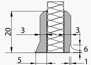
OP20F MET VOET OP20RB MET UITSPARING
