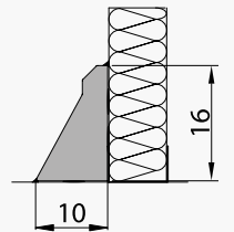
OP20F MET VOET OP20RB MET UITSPARING
